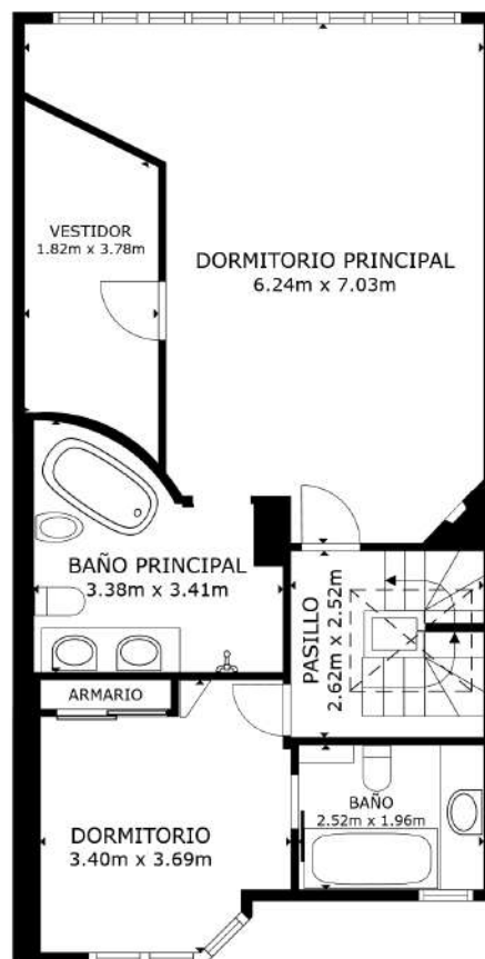
PLANTA 2
